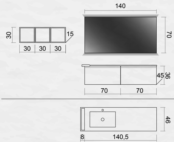
Encimera KATRINA seno izquierda con toallero izquierda y orificio grifo. KATRINA countertop left displaced breast with towel rack left and tap hole. / Plan KATRINA déplacé sein gauche avec porte-serviettes gauche et le trou du robinet.
