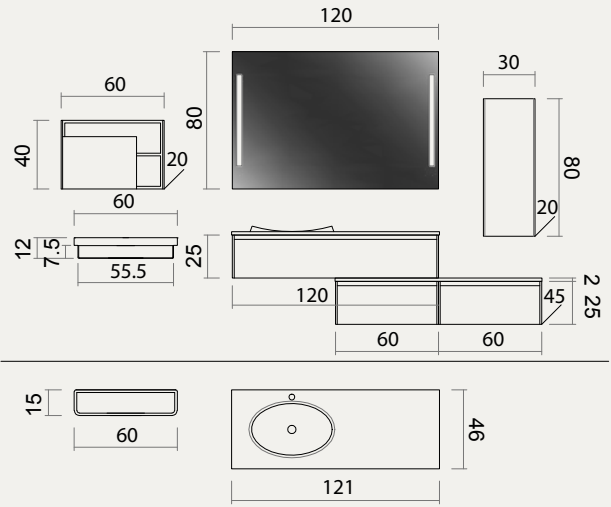
Espejo HOLLY 120 ancho x 80 alto. / HOLLY mirror 120 width x 80 height. / Miroir HOLLY largeur 120 x hauteur 80. Encimera AMARA 121 ancho x 46cm seno izquierda con orificio para grifo. / AMARA countertop 121 x 46cm left displaced breast withn tap hole . / Plan AMARA 121 x 46cm déplacé sein gauche avec le trou du robinet.
