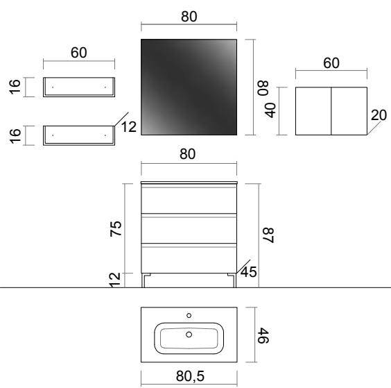
Estante SMILE melamínico diseño 02 Cream. / SMILE shelf melamine design 02 Cream. / Étagère SMILE mélamine design 02 Cream. Espejo TECHNO. / TECHNO mirror. / Miroir TECHNO. Aplique LANDA pequeño a marco. / LANDA wall lamp small to frame. / Applique LANDA petit à cadre.
