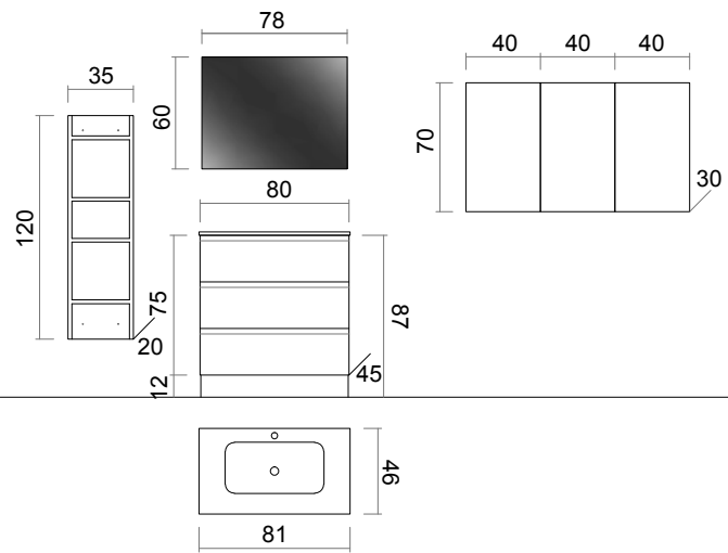
Mueble lavabo VELICE Roble Rústico Envejecido. Zócalo Nieve Mate. / Washbasin furniture VELICE Rustic Aged Oak. Nieve matt Plinth. / Meuble vasque VELICE Chaîne Rustico Vieilli. Zocalo Nieve mat.
