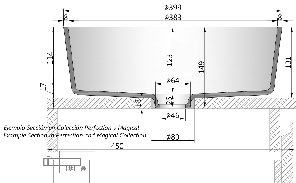
SECCIÓN A-A' SECTION A-A'
