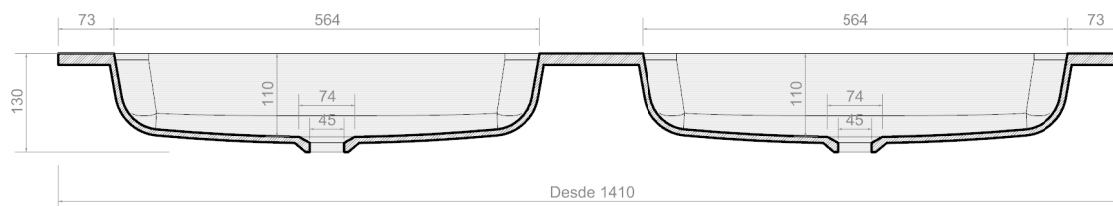
SECCIÓN A-A' SECTION A-A'
