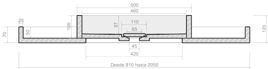
SECCIÓN A-A' SECTION A-A'
