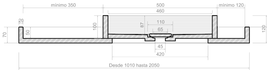
SECCIÓN A-A' SECTION A-A'
