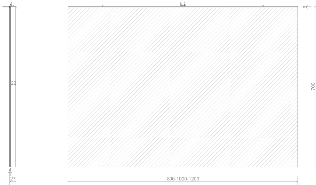
PERFIL
