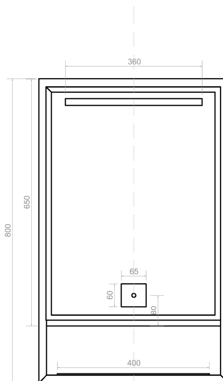
ALZADO TRASERA
